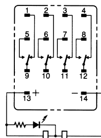
MY4(Z)N1/MY4(Z)IN1 (только модели для пост. тока)
