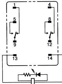
MY2N/MY2IN (модели для перем. тока)
