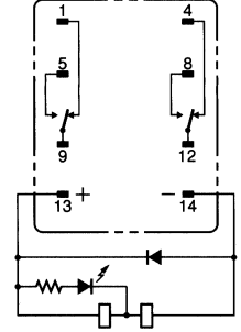
MY4(Z)N-D/MY4(Z)IN-D2 (только модели для пост. тока)
