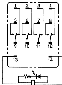
MY4(Z)N-CR/MY4(Z)IN-CR (только модели для перем. тока)
