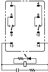
MY4(Z)N/MY4(Z)IN (модели для перем. тока)
