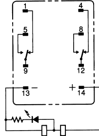
MY2N/MY2IN (модели для пост. тока)
